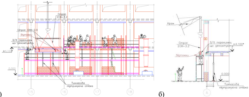
Рис. 2. Схема виконання робіт з розбирання ділянок зовнішніх стін та демонтаж перемичок (проектний варіант): а-вид з боку головного фасаду; б- поперечний розріз
